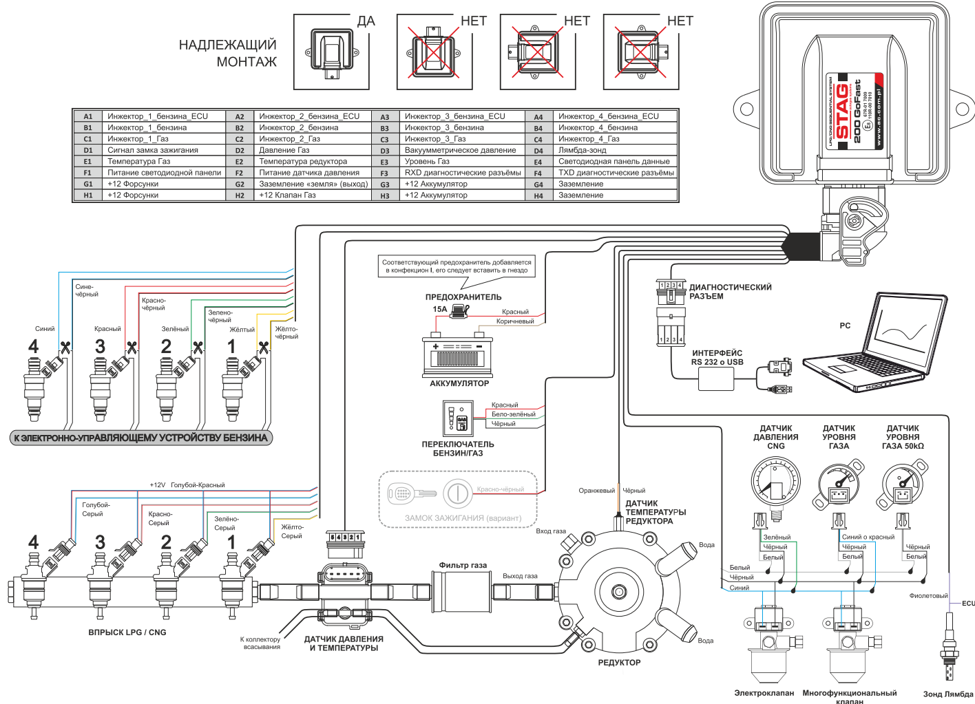
Рис 1. Схема подключения STAG 200 GoFast к автомобильному ГБО.
