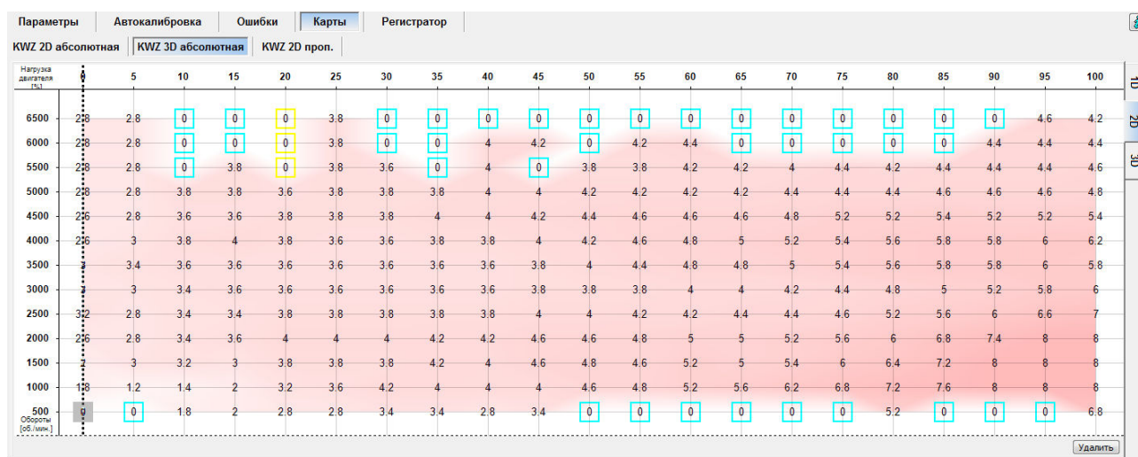
Рис. 22. Результат работы автоадаптации на абсолютной карте 3D.
