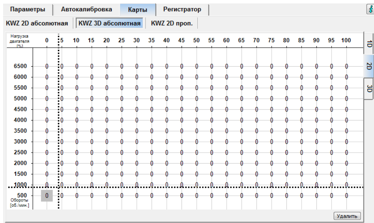
Рис. 17. Вид абсолютной карты KWZ 3D.
