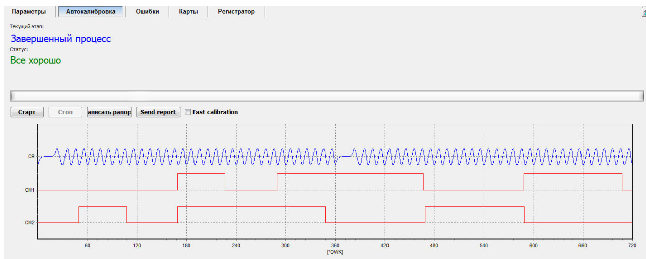
Рис. 11. Вид окна с результатом автокалибровки.
