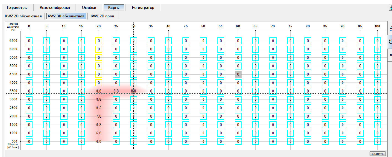
Рис. 21. Абсолютная карта 3D после сбора основных пунктов главного столбца вариатора.
