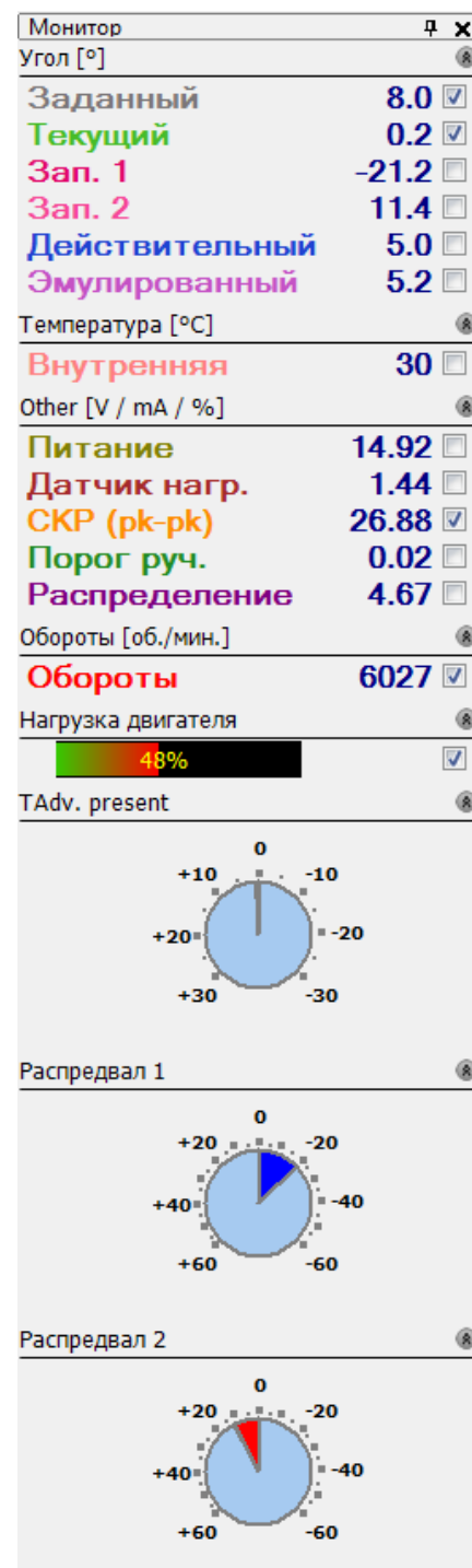
Рис.9. Вид окна «Монитор».
