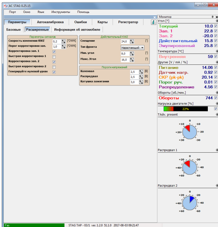
Рис. 5. Вид окна «Дополнительные параметры».
