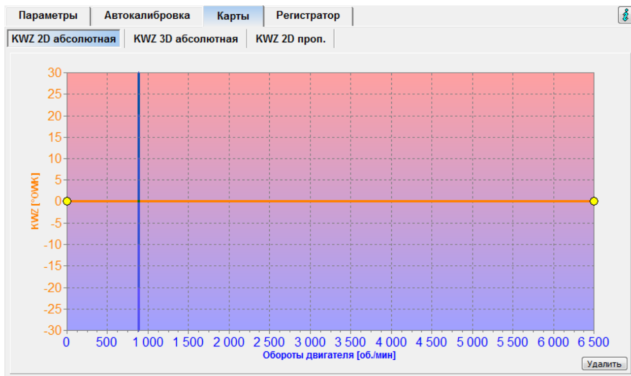
Рис. 15. Вид абсолютной карты угла опережения зажигания 2D.
