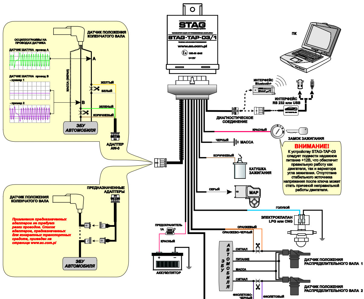
Рис. 2. Схема подключения STAG-TAP-03/1 (индуктивный датчик положения коленчатого вала).
