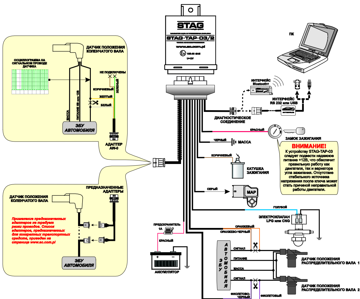
Рис. 3. Схема подключения STAG-TAP-03/2 (датчик Холла или оптический датчик положения коленчатого вала).
