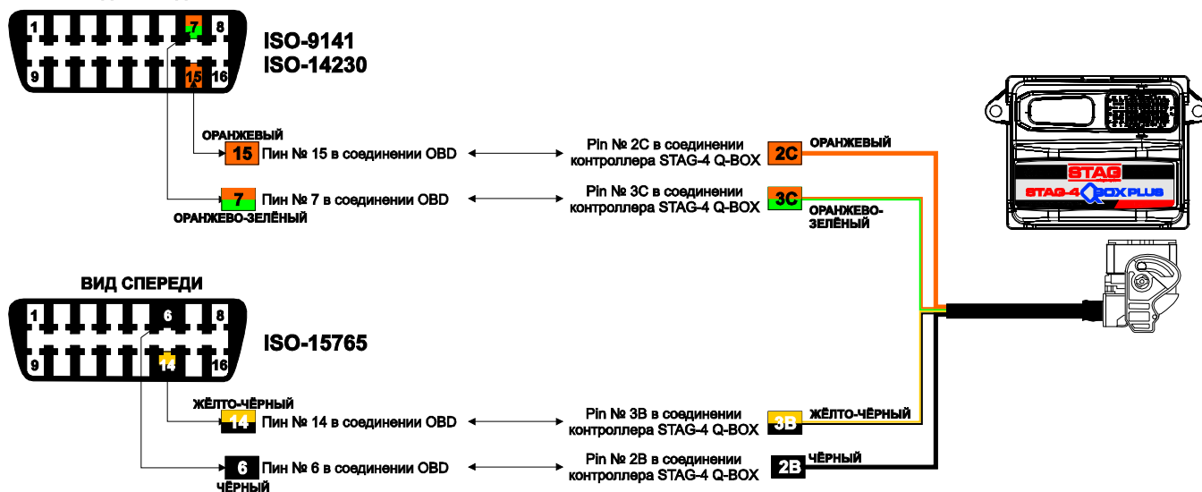
Рисунок 3 Схема подключения STAG-4 QBOX / QNEXT / QMAX PLUS в разъем OBD.
