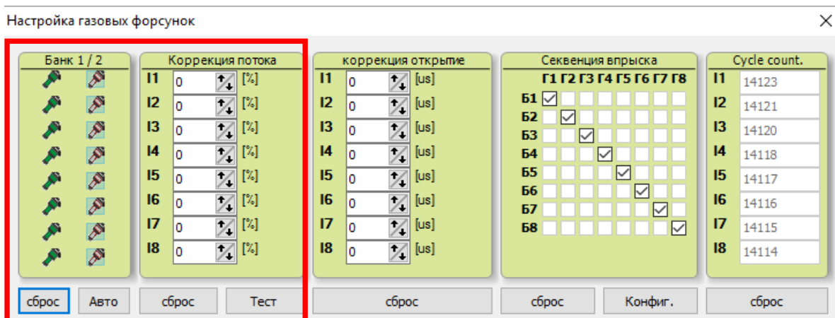
Рисунок 51 Присвоение газовых форсунок соответствующему банку.
