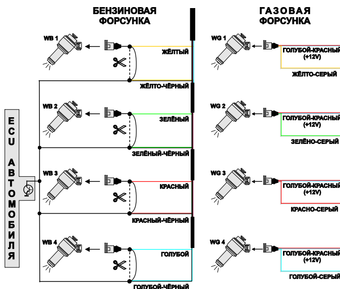
Рисунок 12 Схема подключения к автомобильному оборудованию при управлении «full group».
