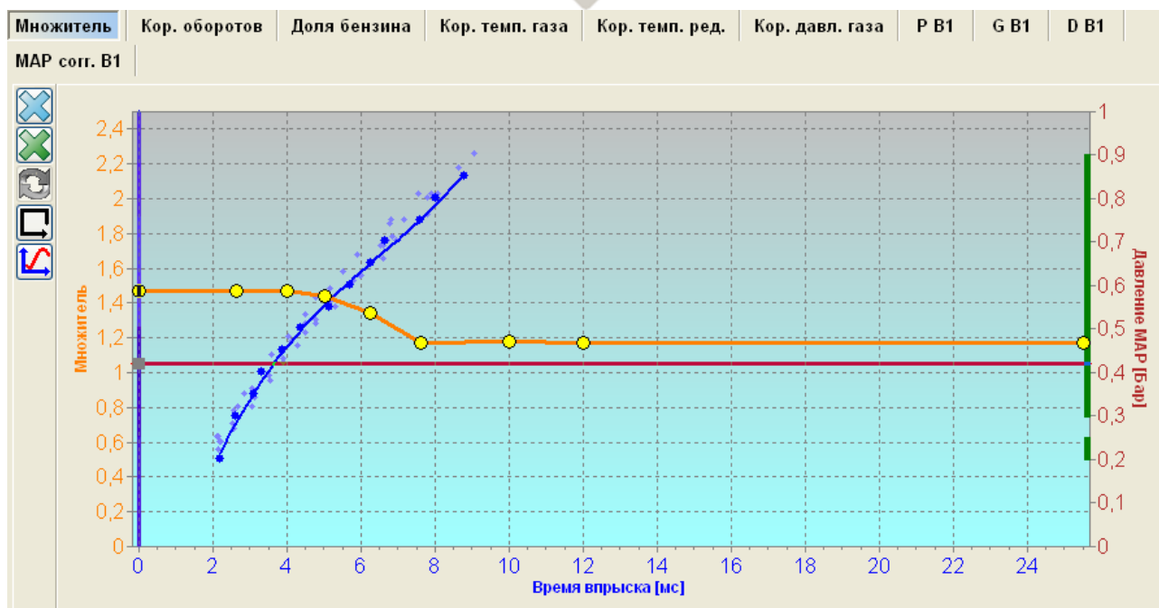
Рисунок 35 Карта множителя. Действие функции «Подгонка множителя».
