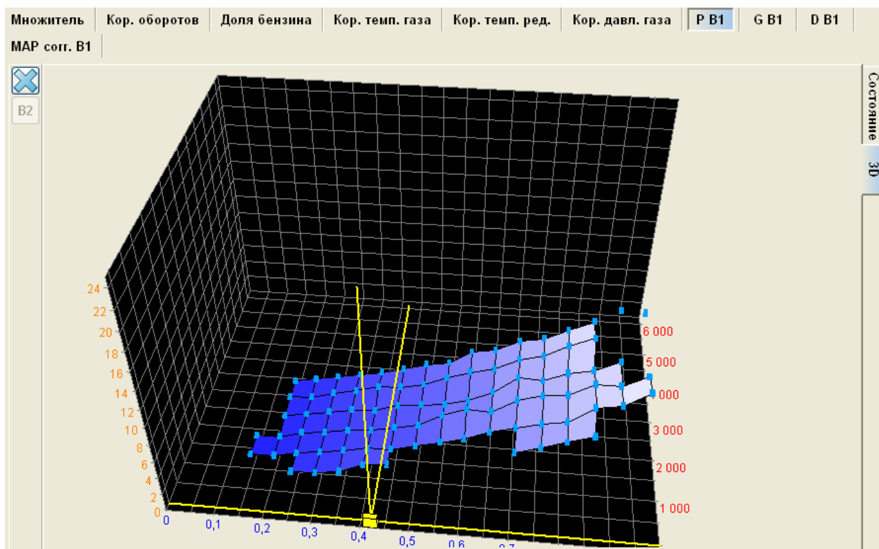
Рисунок 42 Состояние сбора бензиновой карты.
